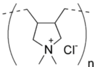
Figura 1 - Estrutura química do Poly Dadmac
