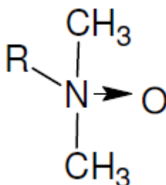
Figura 1 - Estrutura geral de uma amina oxida
